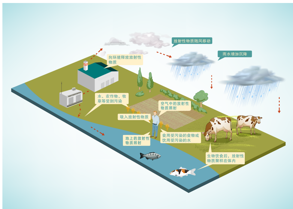
图 1.3-1 辐射照射途径示意图
