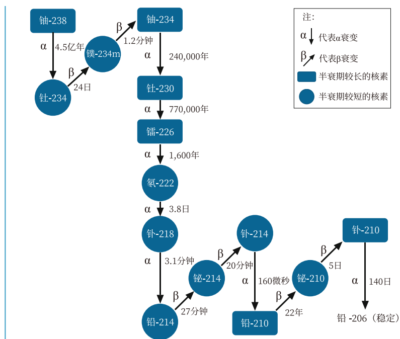
■ 图1.1-2 铀-238主要衰变系列示意图
