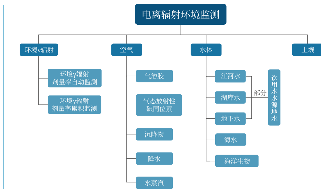
图 2.2-1 电离辐射环境监测对象示意图
