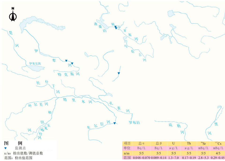
图 3.3.1-9 西北诸河布点和监测结果示意图 (注：西北诸河中镭-226因仪器设备、采样、样品前处理、测量等原因导致数据缺失。)
