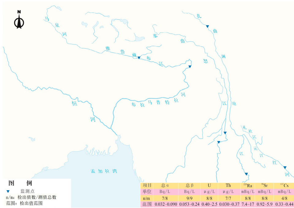
图 3.3.1-10 西南诸河布点和监测结果示意图
