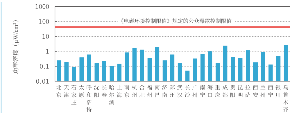
图 3.5-2 环境电磁辐射水平
