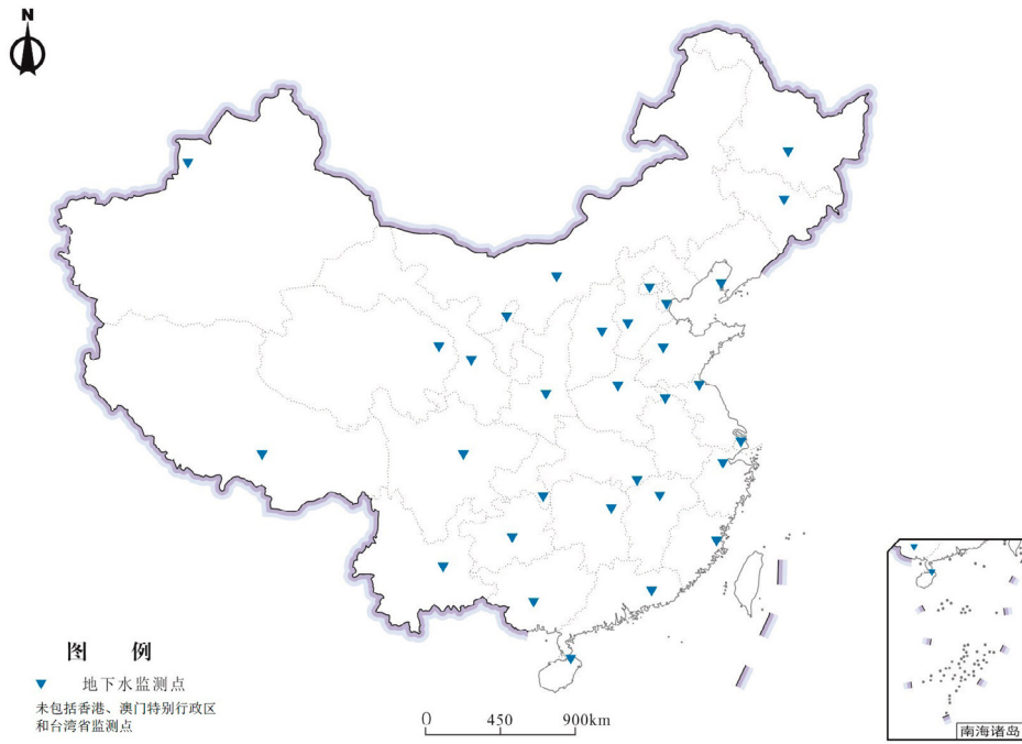
图 3.3.4-1 地下水布点示意图
