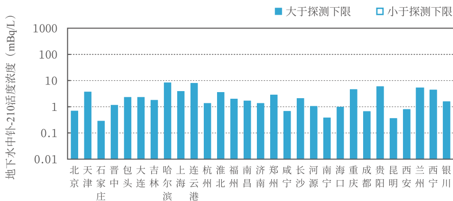
图 3.3.4-7 地下水中钋-210活度浓度
