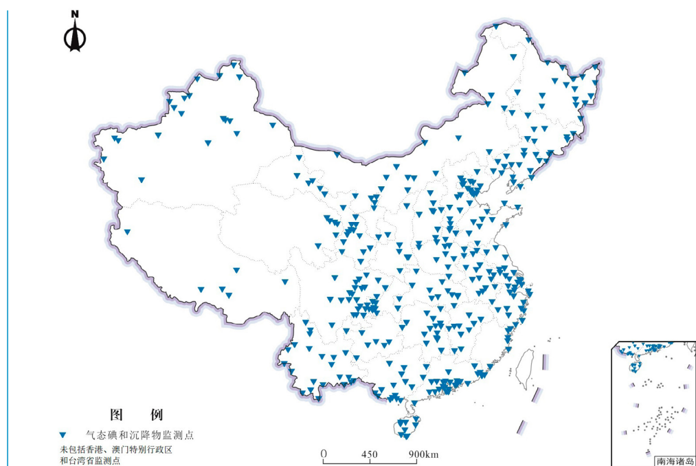
■ 图 3.2.3-1 沉降物布点示意图
